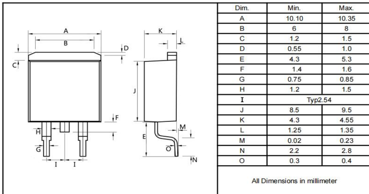
T0-263
